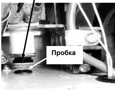
Регулятор минимального давления газа
